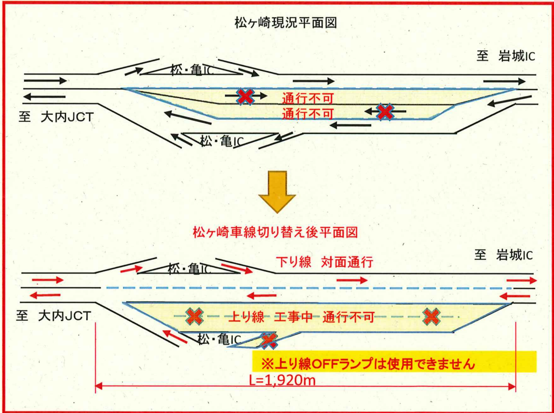
◎車線切り替え後平面図
