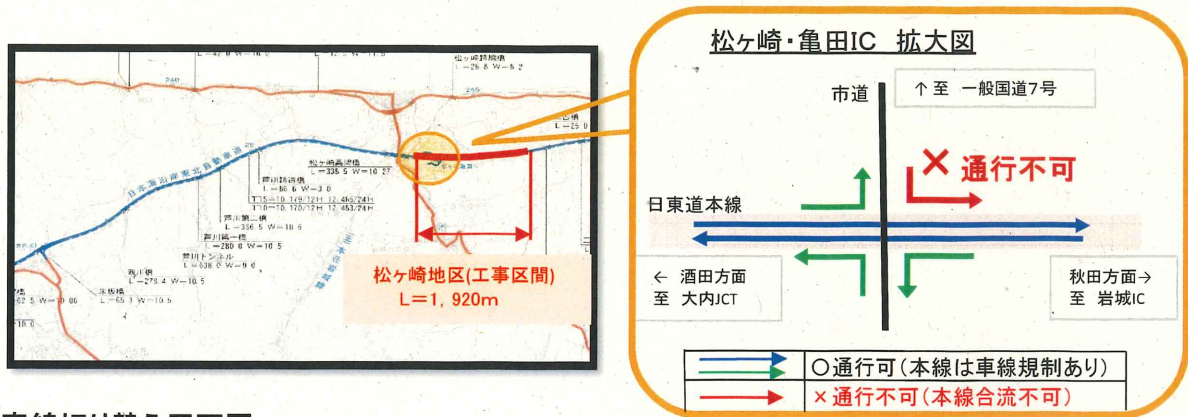
◎車線切り替え平面図
