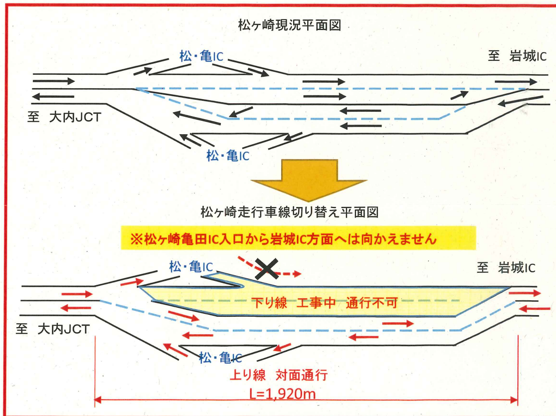
◎車線切り替え平面図
